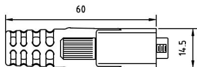
MDRコネクタ
